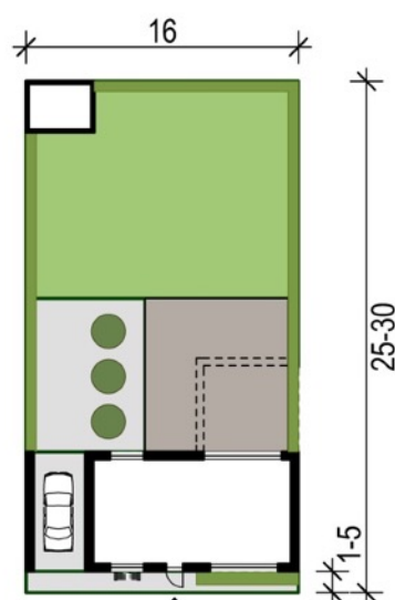
Hustyp 2 1,5 plan 120-150 m 2 - Tomt 400-480 m 2
