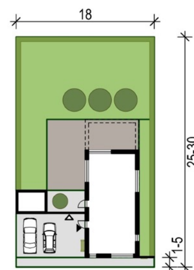
Hustyp 3 1,5 plan 130-150 m 2 - Tomt 400-550 m 2
